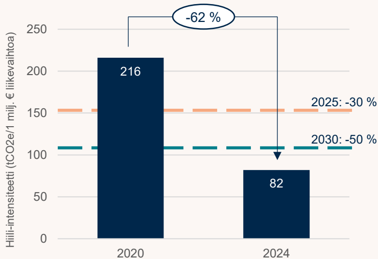
Suorien listattujen osakkeiden hiili-intensiteetti
