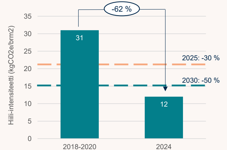
Kotimaisten kiinteistöjen hiili-intensiteetti
