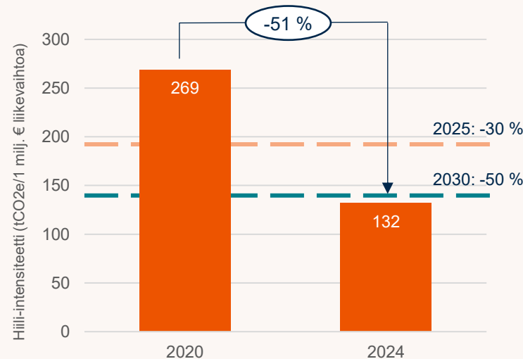
Suorien listattujen yritysten jvk-lainojen hiili-intensiteetti
